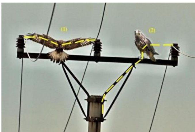
Ilustración 14. Representación de la electrocución de aves.
