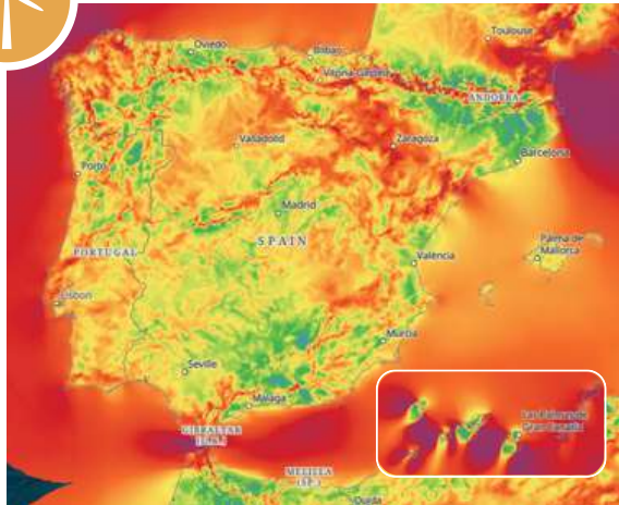
Figura 9. Zonas de recurso eólico y fotovoltaico disponible. Fuente: Global Solar Atlas , Global Wind Atlas .
