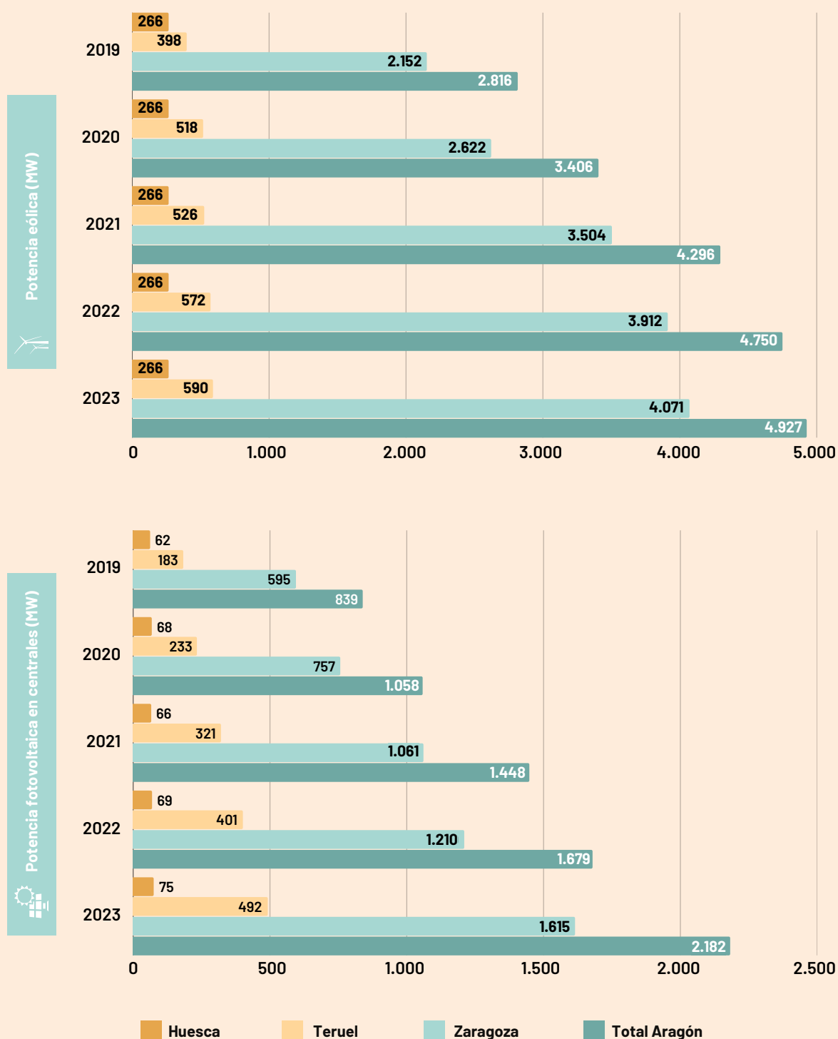
Figura 6. Potencia eólica y fotovoltaica en Aragón y sus provincias de 2019 a 2023.
