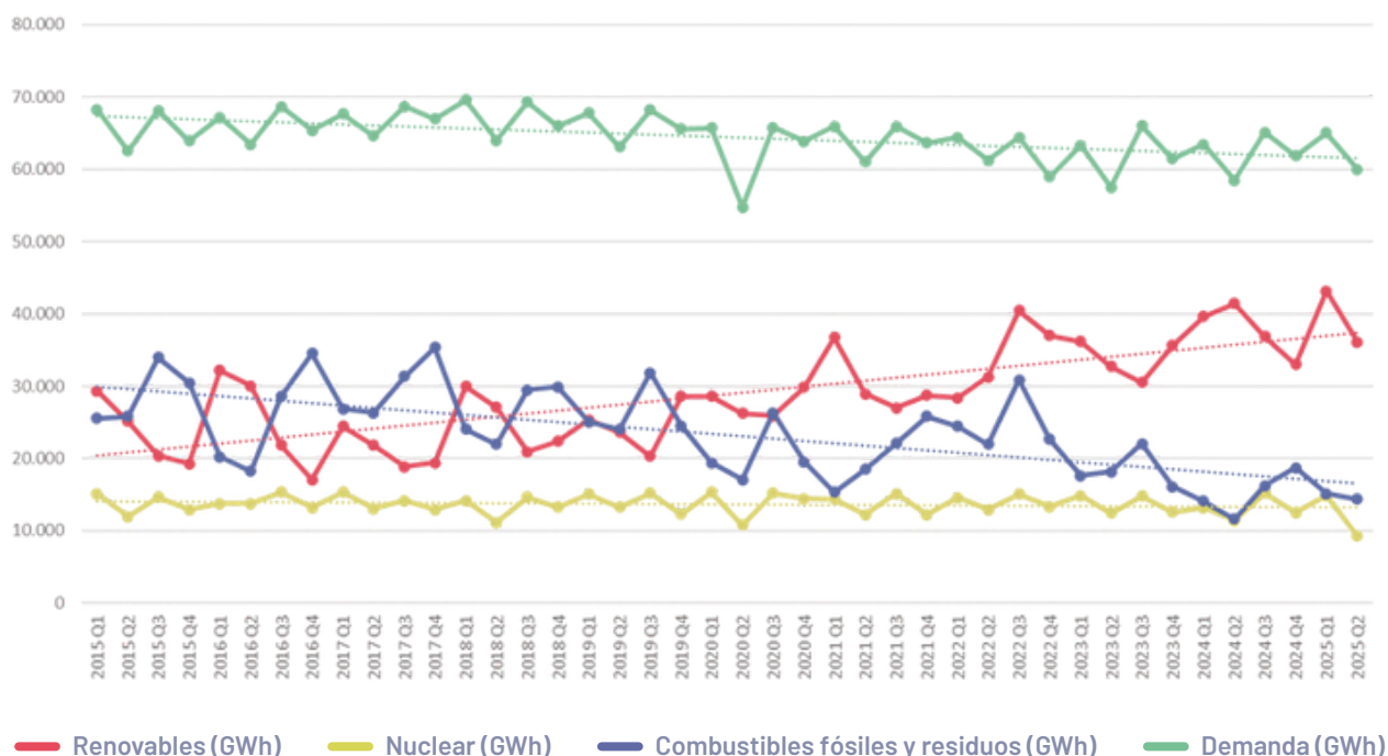
Figura 20. Demanda y generación eléctrica estacional desde 2015 hasta 2025 de nuclear, combustibles fósiles y residuos y renovables.
