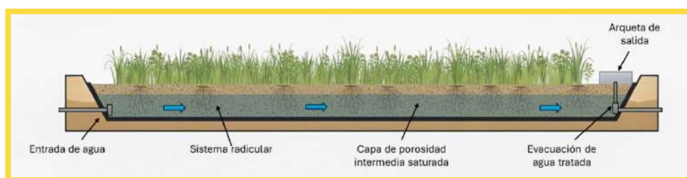
Figura 40. Esquema de humedal de flujo horizontal.
