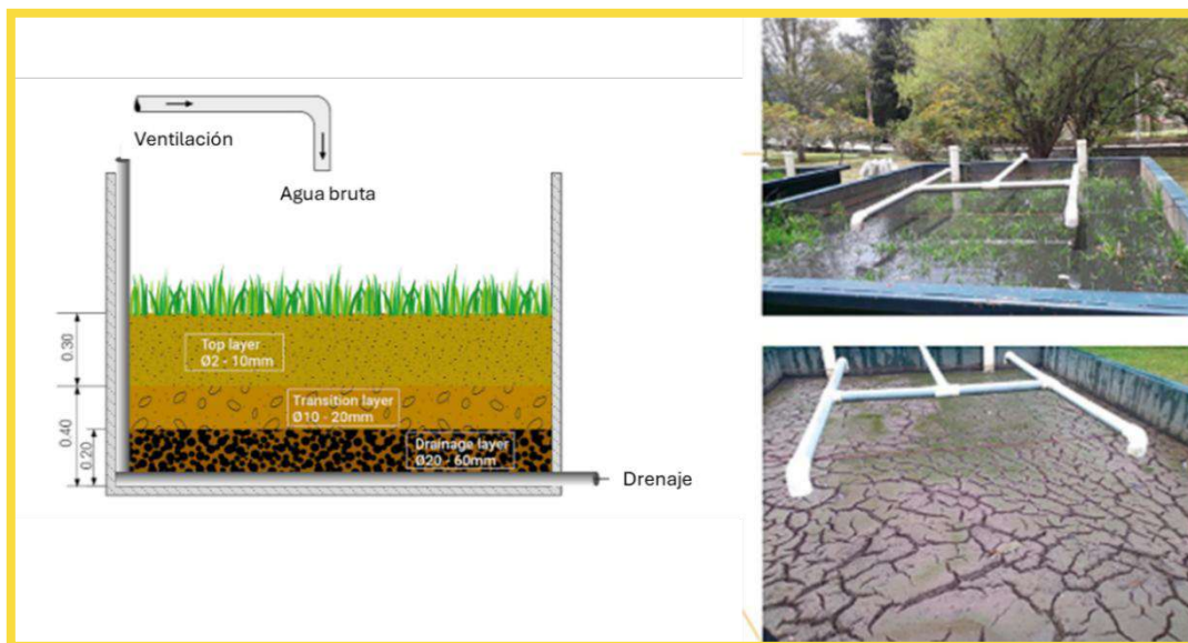
Figura 39. A la izquierda, esquema y capas que presenta el primer humedal. A la derecha, estado del humedal cuando recibe el agua bruta y tras el periodo de reposo y mineralización del fango.
